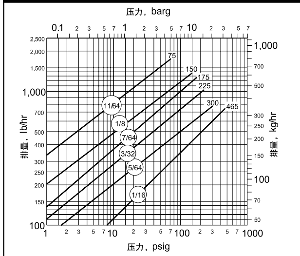
ICS 系列排量图 DN40 (1 1/2")
