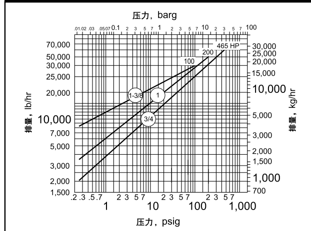
ICS 系列排量图 DN50 (2")
