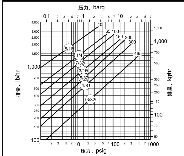
ICS 系列排量图 DN50 (2")
